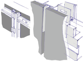
Mechanical clamping / Mechanické kotvení
