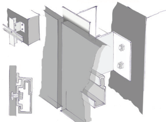
Undercut anchors / Spodní mechanické kotvení
